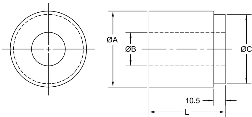
SPACER
