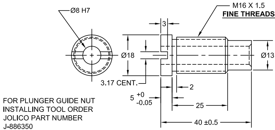
PLUNGER GUIDE NUT
