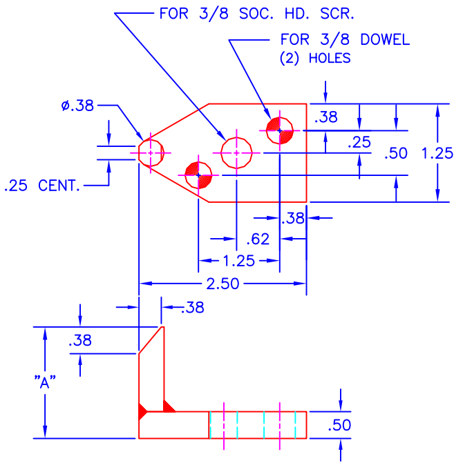
PIN GAGE
