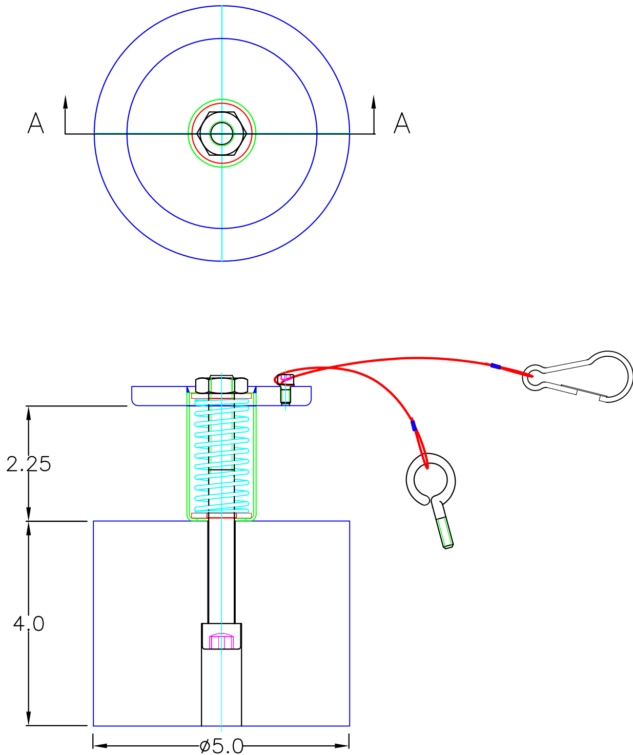
SECTION A-A
